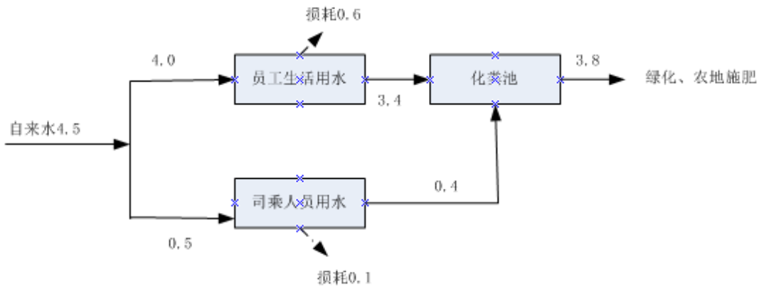
图 1-1 本项目水平衡图 (m 3 /d)
