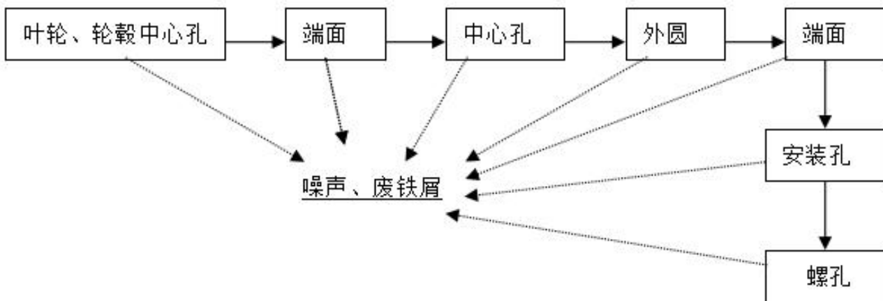
图 2-3 叶轮、轮毂生产流程图
