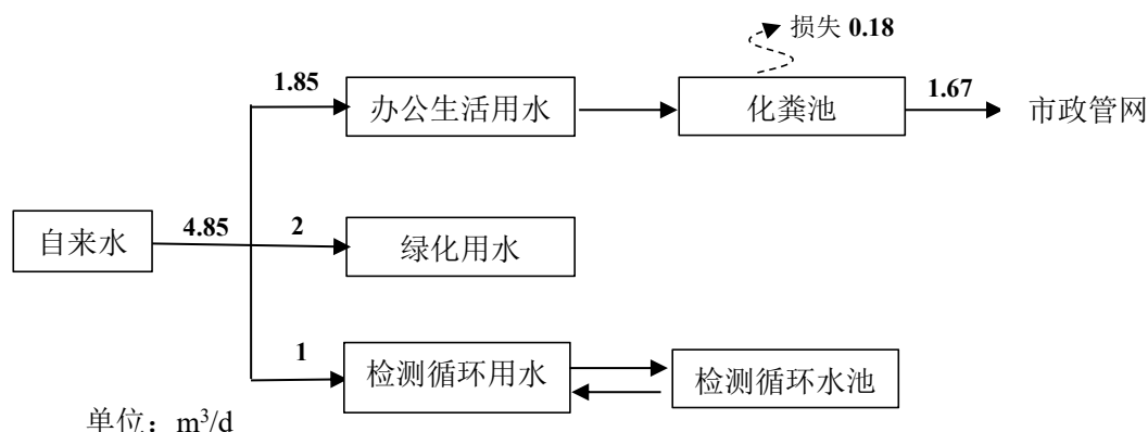
图 2-1 项目运营期水平衡图
