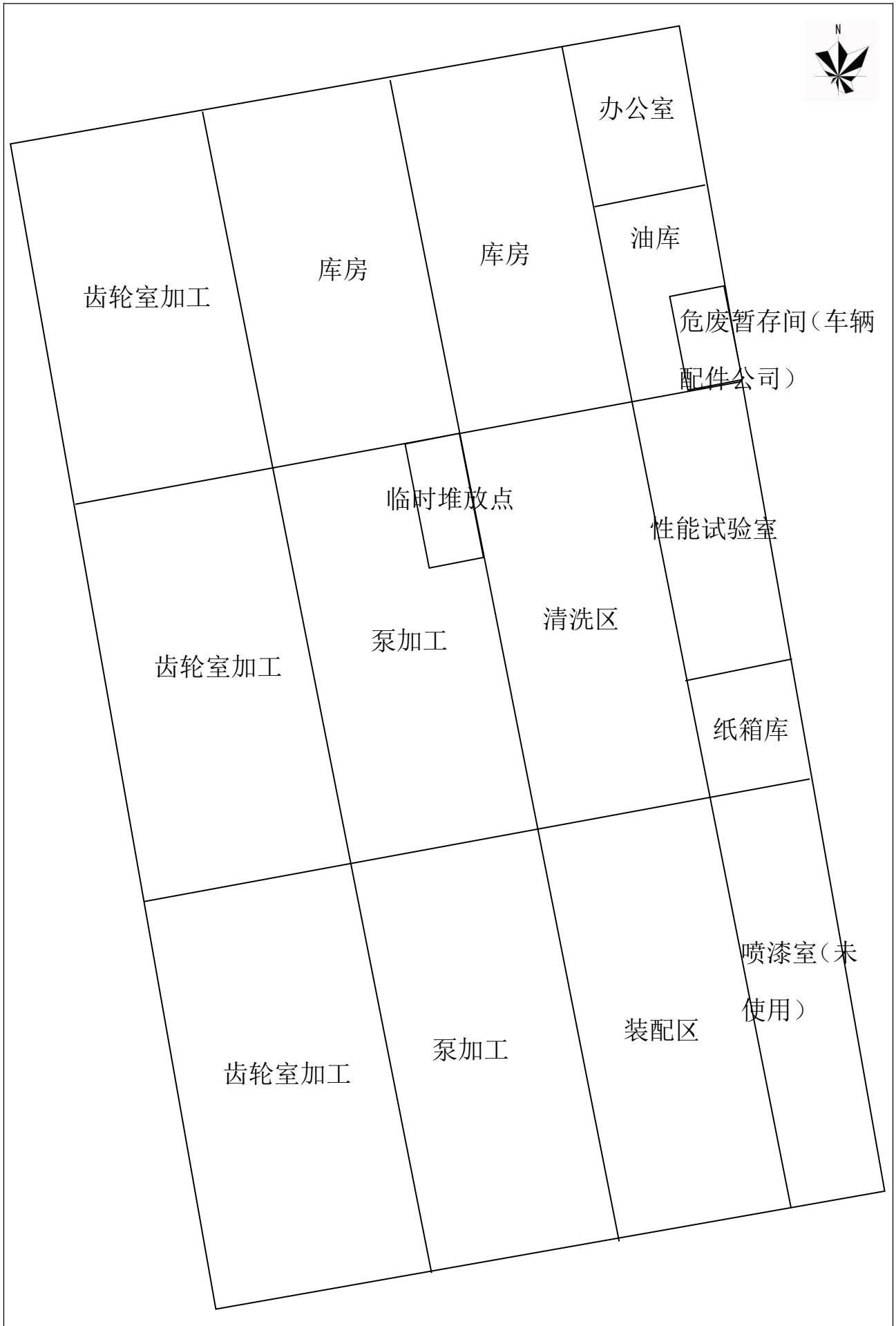
附图 4 项目生产车间平面布置图
