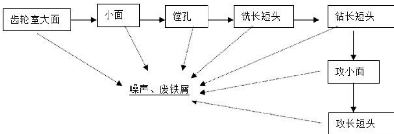
图 2-5 齿轮室生产流程图
