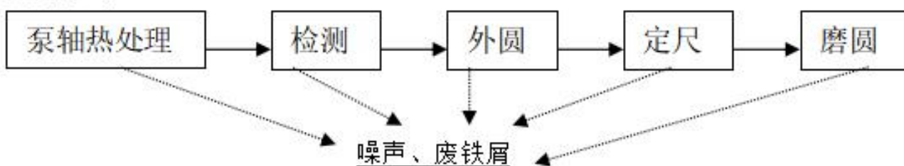
图 2-4 泵轴生产流程图
